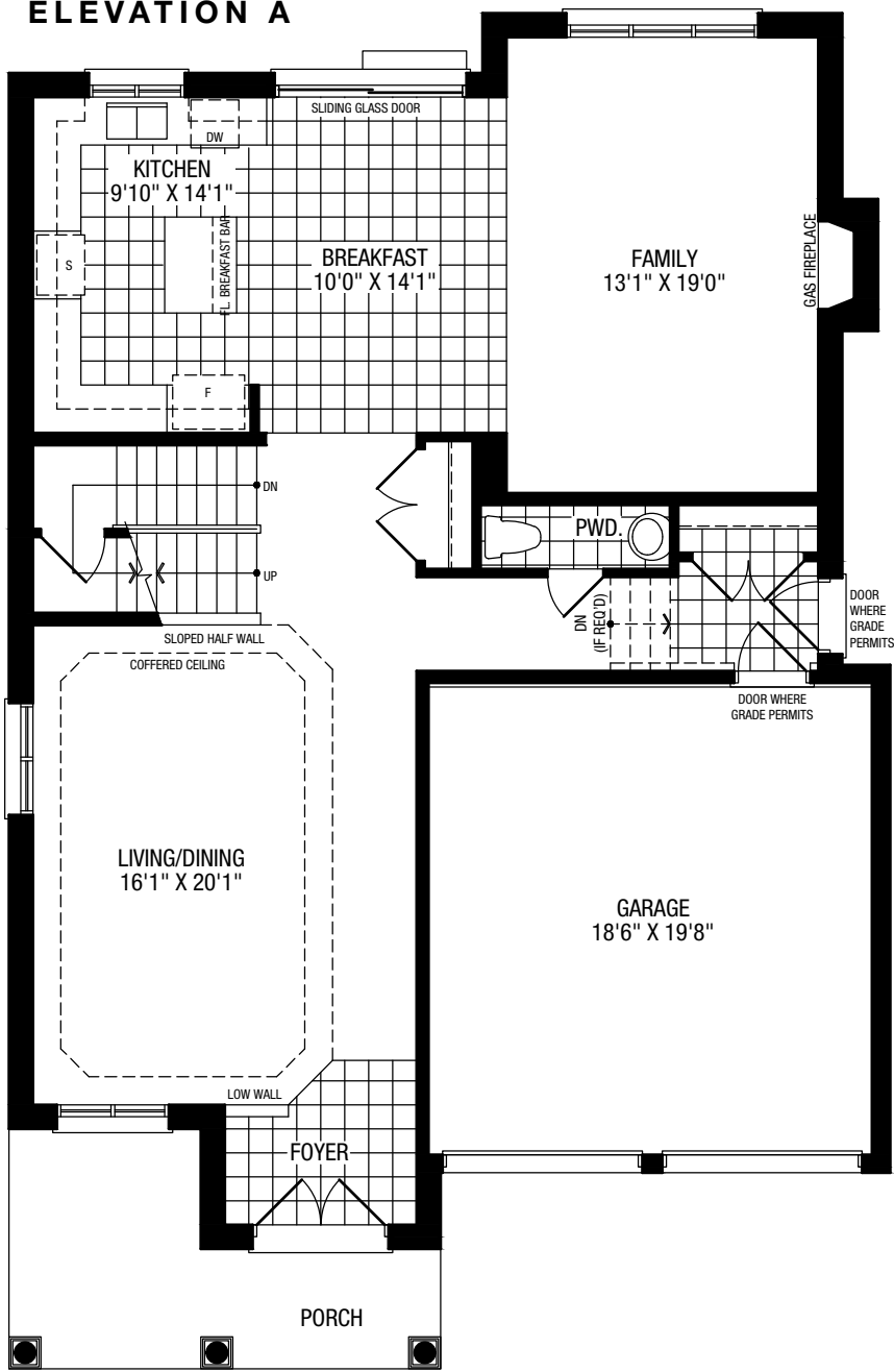
ELEVATION A
